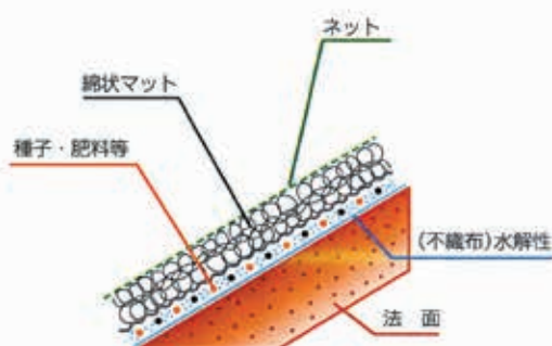
テンテックスフィルターの構造
