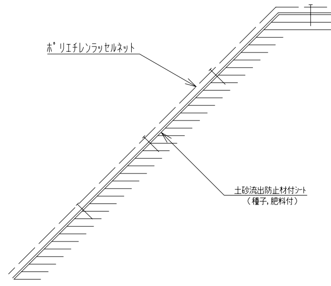
施工断面図 (S=1/20)
