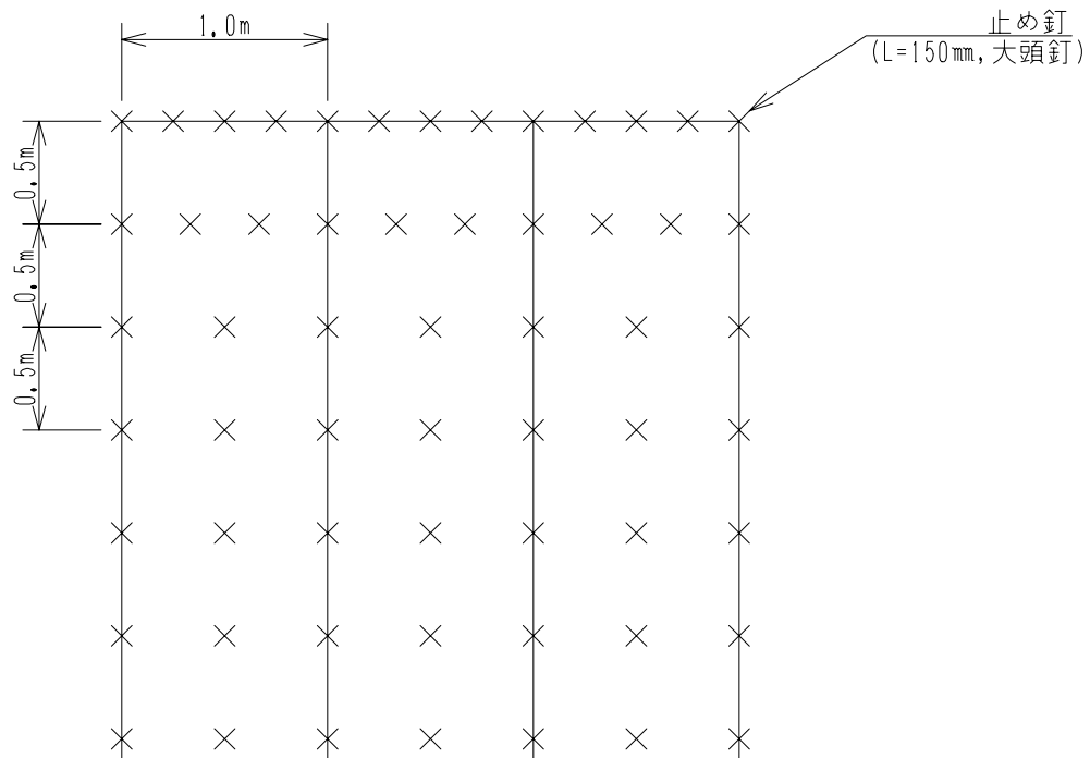
アンカー打設図 (S=1/40)
