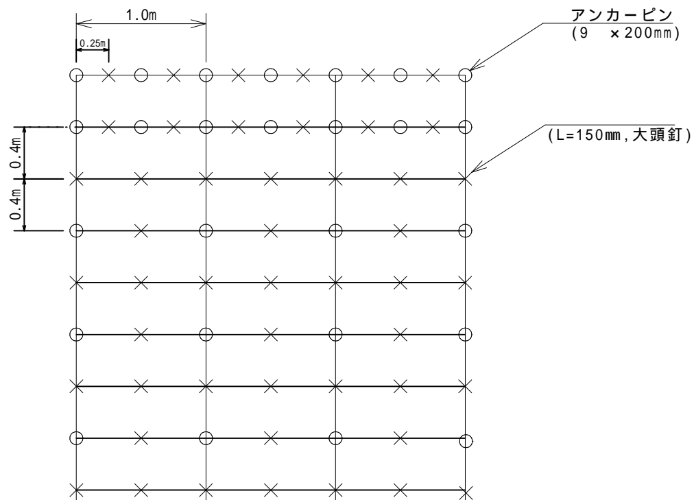
アンカー打設図 (S=1/40)
