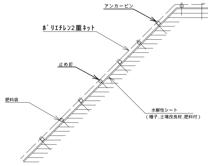
施工断面図 (S=1/40)
