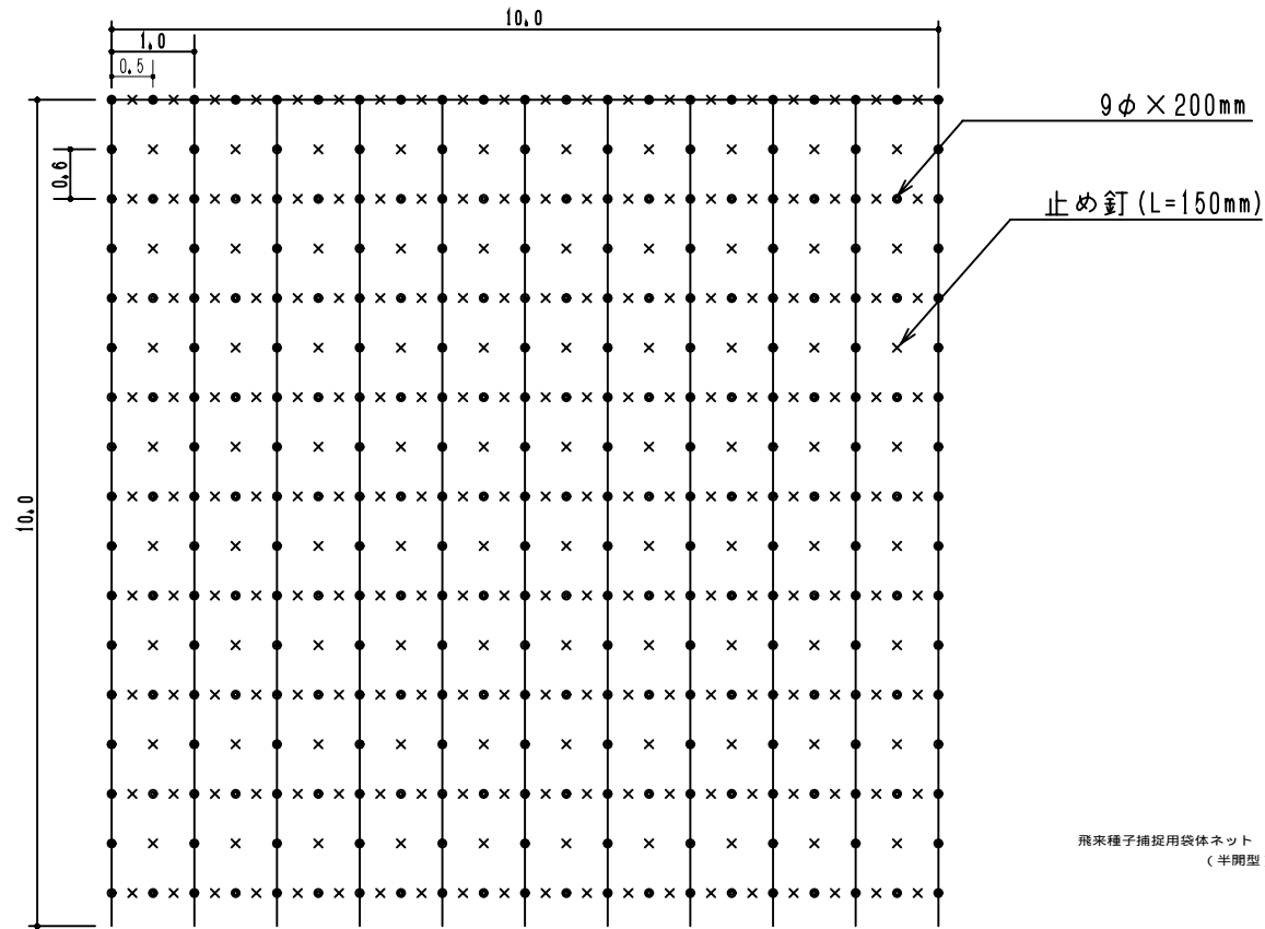
標準打設図
