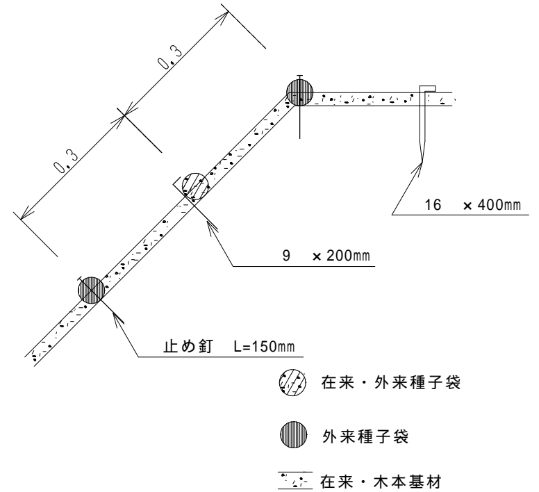
断面図
