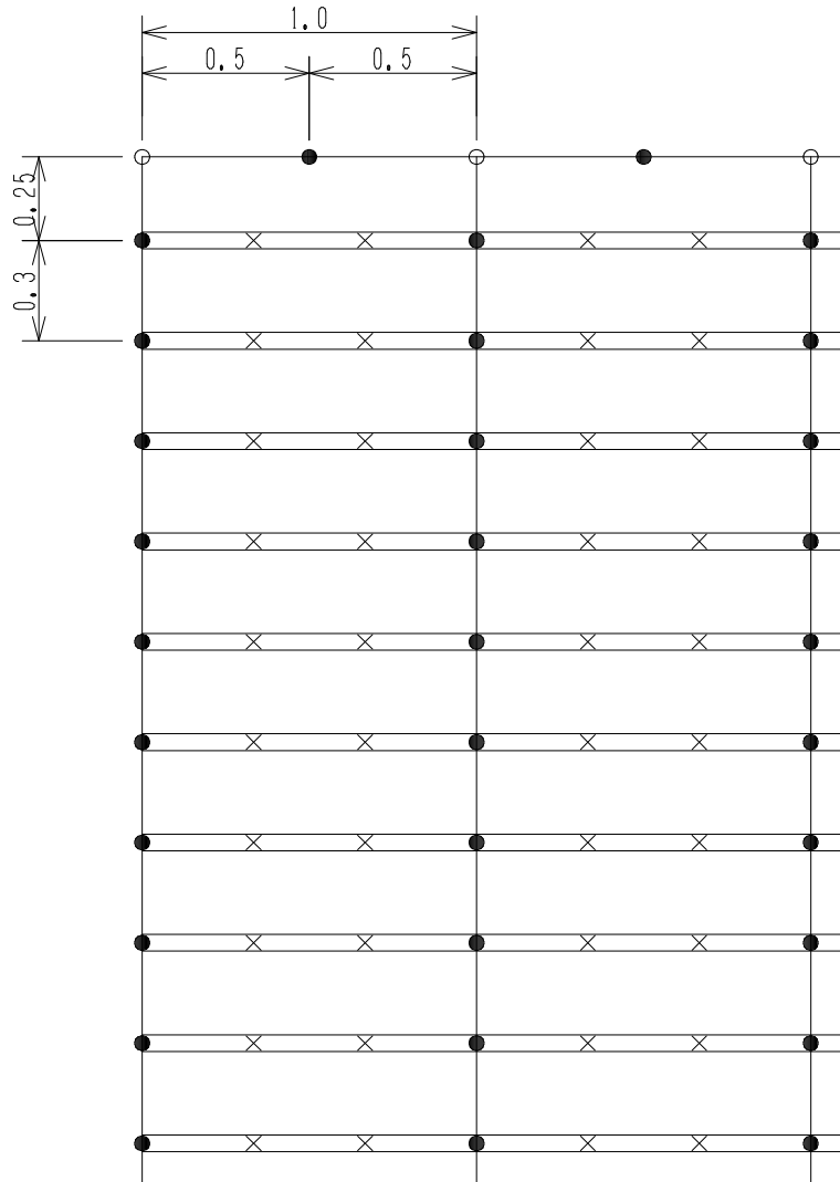
標準打設図
