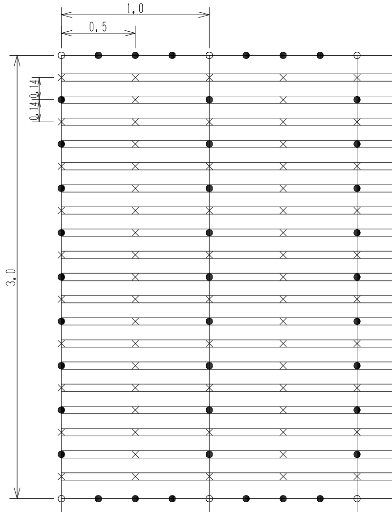
標準打設図
