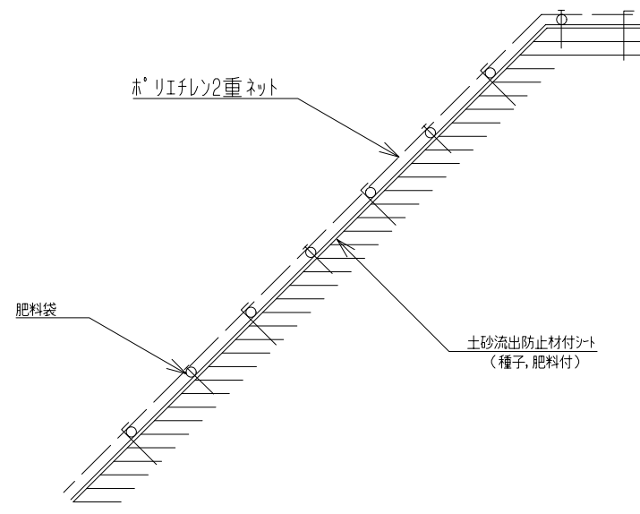
施工断面図 (S=1/40)
