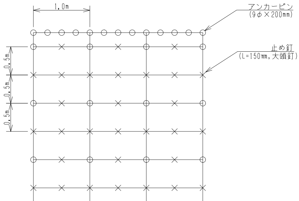
アンカー打設図 (S=1/40)
